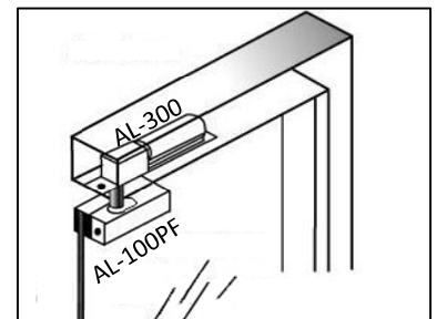
Bracket Contra-pistón AL-100PF (Instalación puerta de vidrio sin marco)
