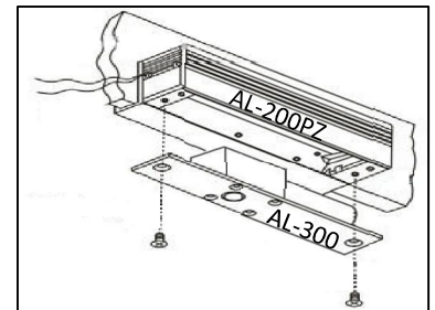
Bracket Pistón AL-200PZ (Instalación puerta de vidrio sin marco)
